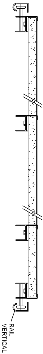
COUPE A-A
